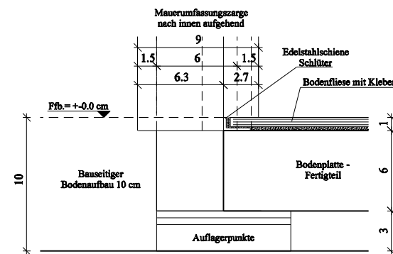
SCHWELLENDetail M 1:2
