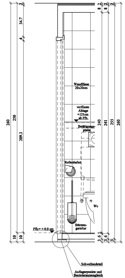
SCHNITT TÜR M 1:10
